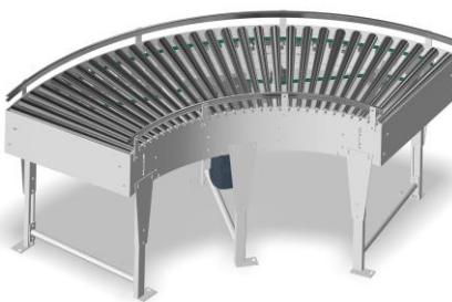
Convoyeur courbe (libre ou motorisé)
